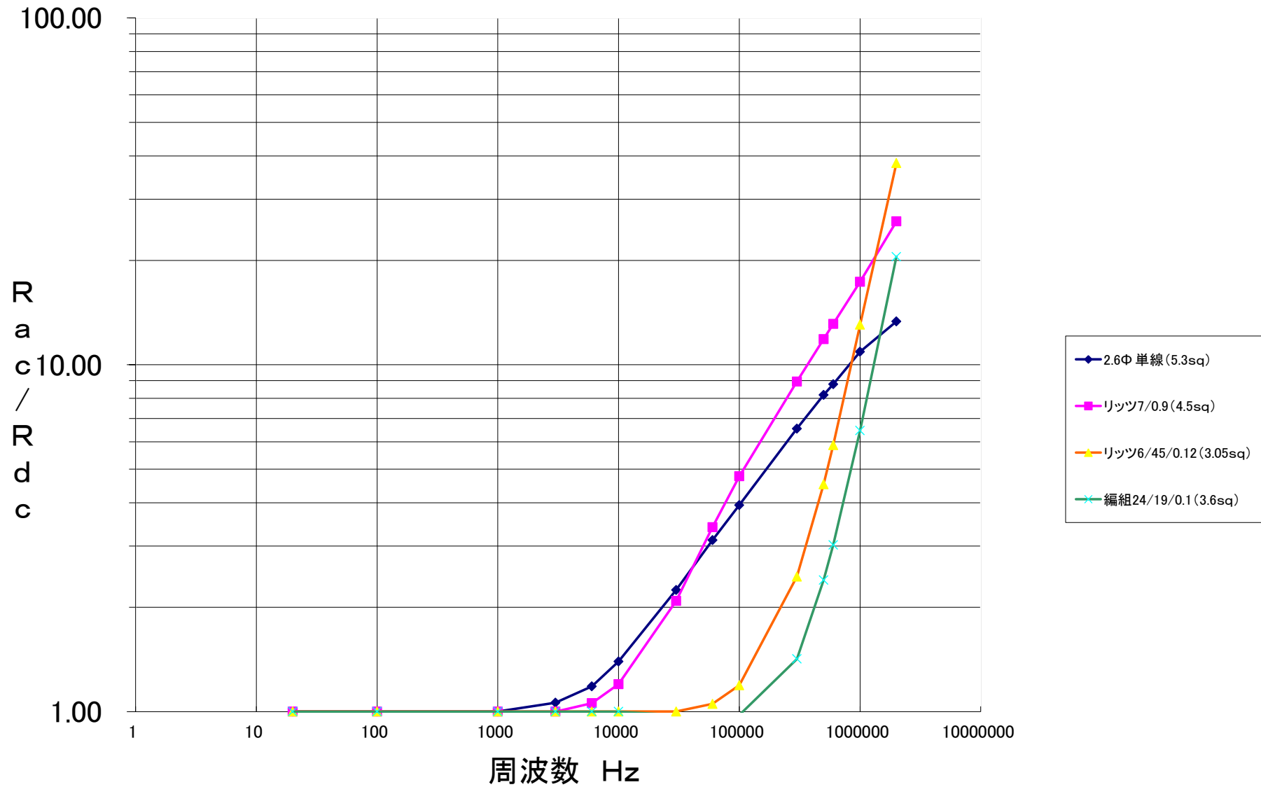
単線と各種撚線の高周波特性比較(3~5sqmm太線)
